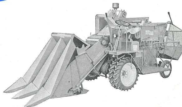
Mietitrebbia completa dell'apparecchiatura per la mietisgranatura del mais
