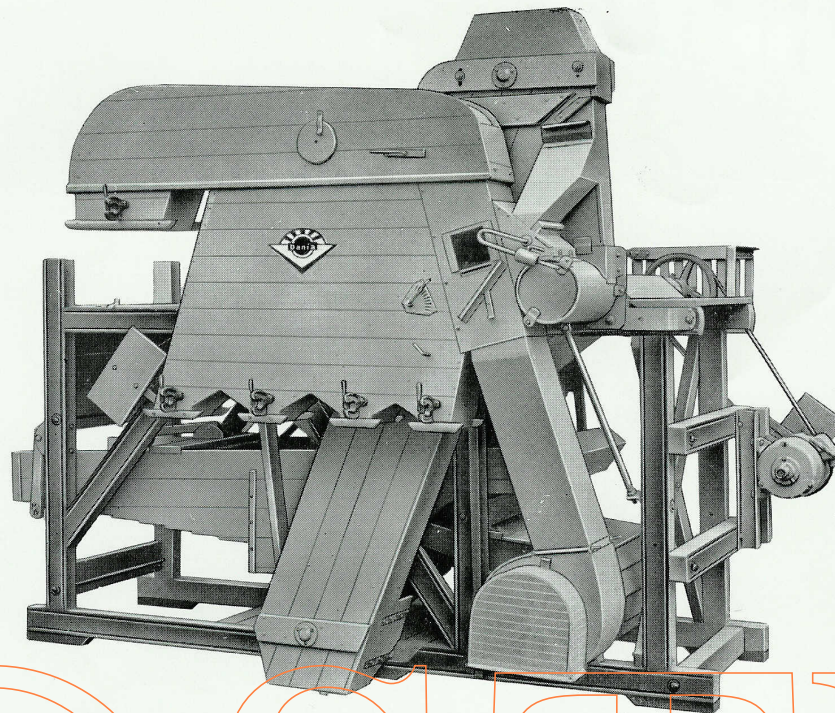
Set fra Udløbssiden med 3 HK Elmotor.
