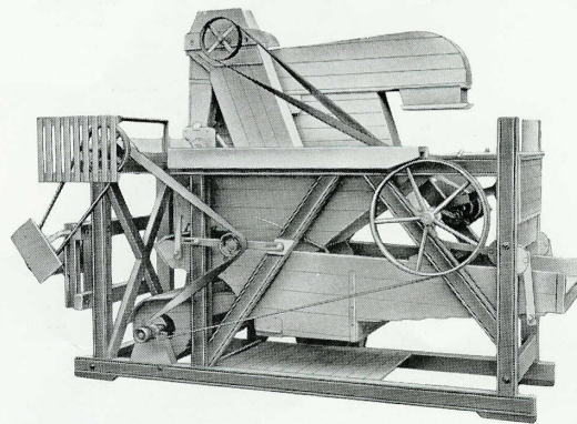
Set fra Renskivesiden.
